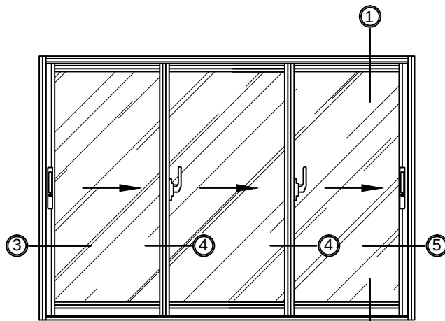
CỬA LÙA 3 CÁNH KHUNG KÍNH HỘP 16-20MM
