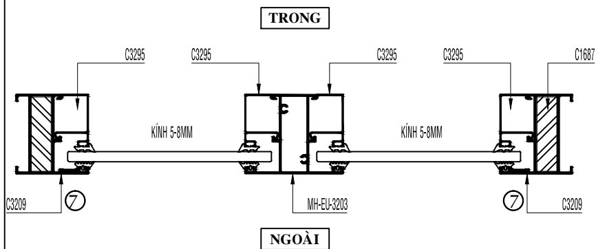
MẶT CẮT NGANG FIX CỐ ĐỊNH
