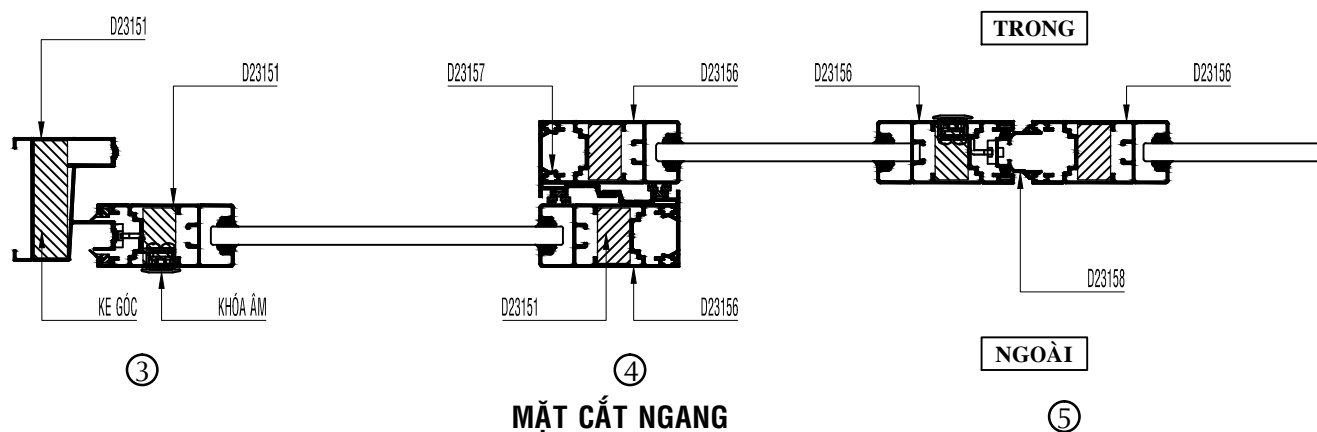
KẾT HỢP CỬA BẬT
