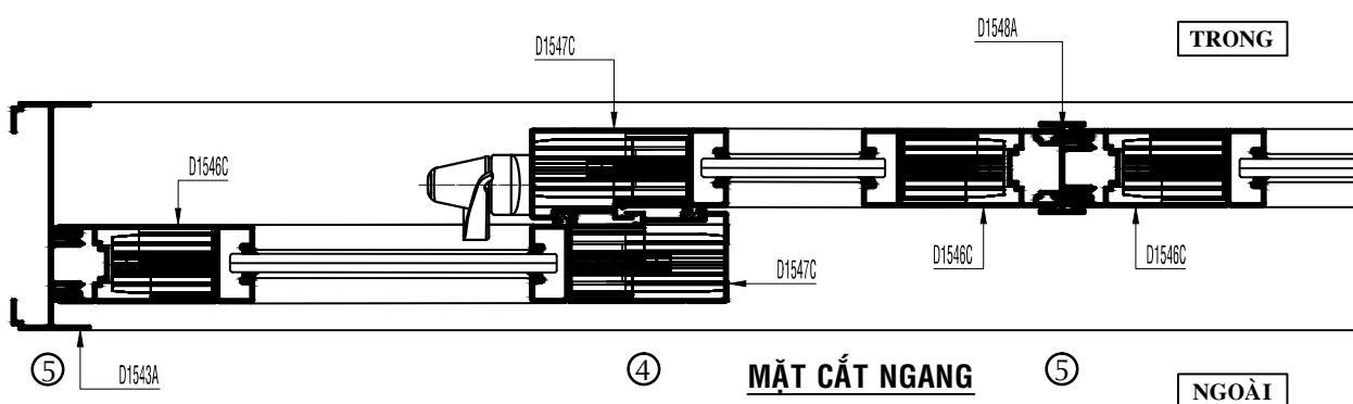
CỬA LÙA 4 CÁNH ( HƯỚNG NHÌN BÊN NGOÀI VÀO )
