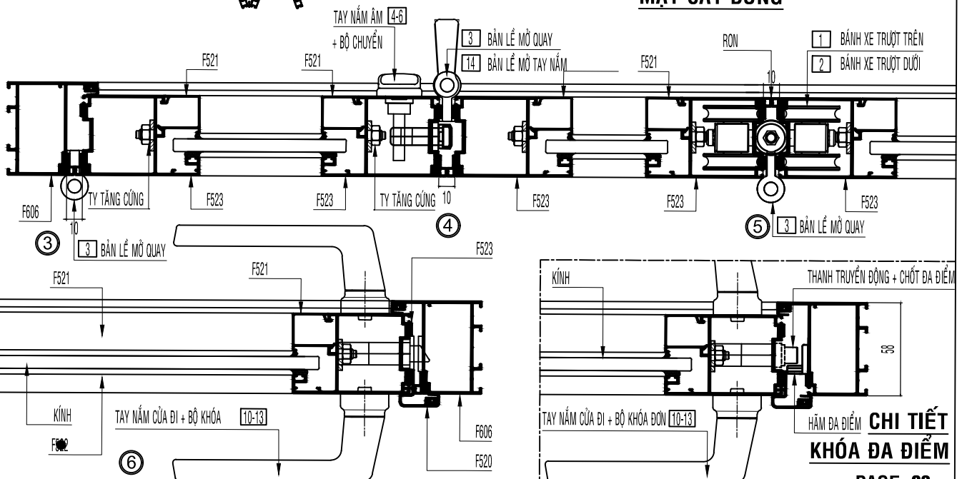
MẶT CẮT ĐỨNG
