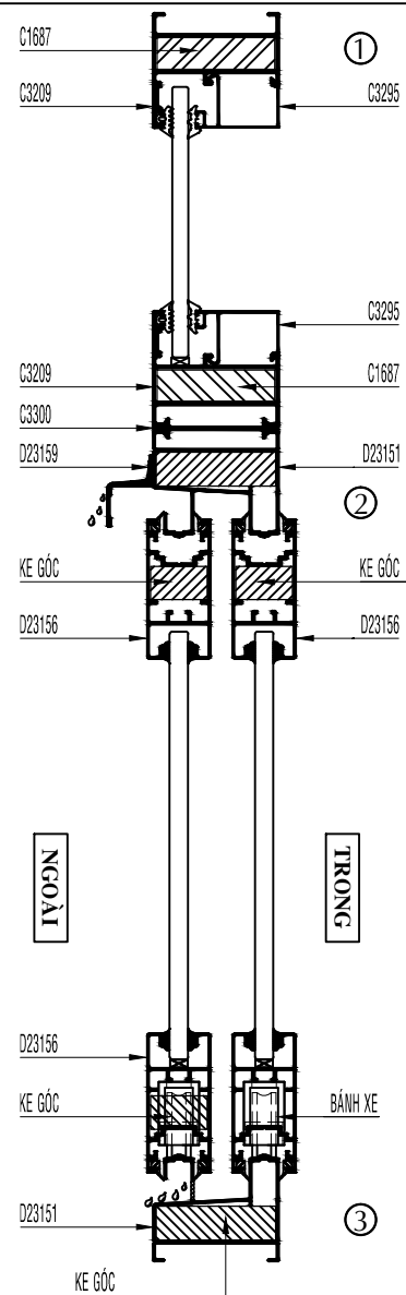
MẶT CẮT ĐỨNG
