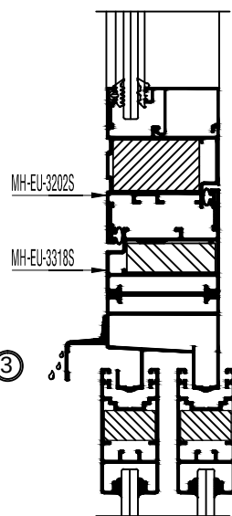
KẾT HỢP CỬA BẬT
