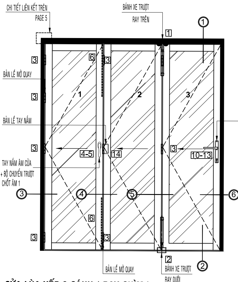
CỬA LÙA XẾP 3 CÁNH ( RAY CHÌM ) HƯỚNG NHÌN : BÊN NGOÀI
