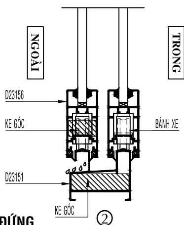
MẶT CẮT ĐỨNG ( KÍNH HỘP )
