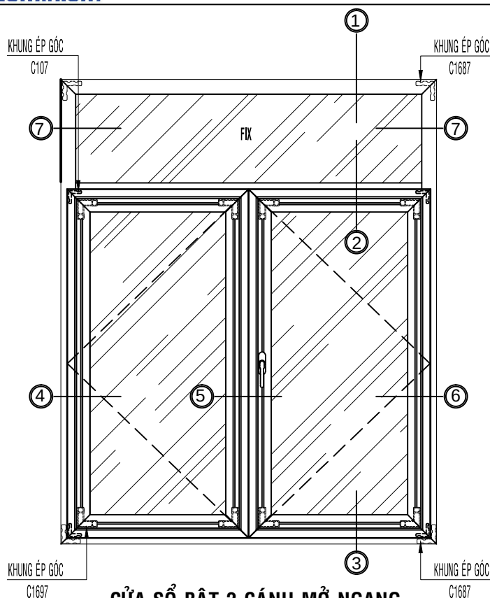
CỬA SỔ BẬT 2 CÁNH MỞ NGANG ( HƯỚNG NHÌN BÊN NGOÀI VÀO )
