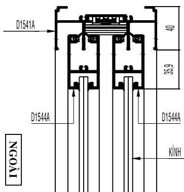
① MẶT CẮT ĐỨNG
