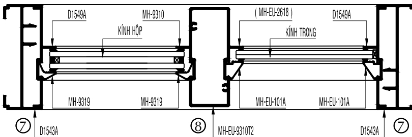
MẶT CẮT NGANG FIX CỐ ĐỊNH
