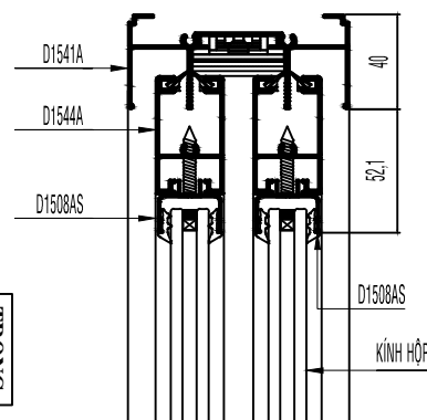
MẶT CẮT ĐỨNG ( KÍNH HỘP )
