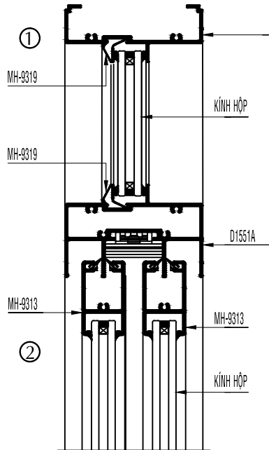
MẶT CẮT ĐỨNG KÍNH HỘP
