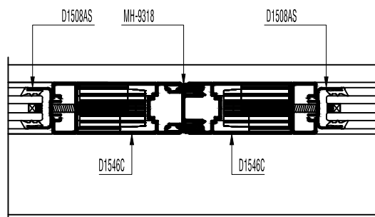
MẶT CẮT NGANG KÍNH HỘP 16-20MM KẾT HỢP
