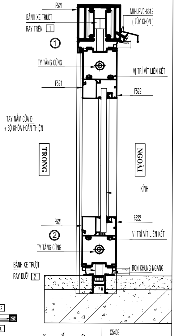
MẶT CẮT ĐỨNG
